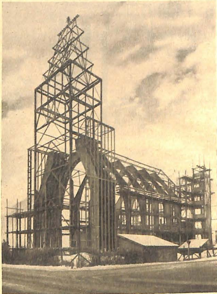
STAHLSCHELETT DES NEUBAUES DER KIRCHE IN DONAWITZ
